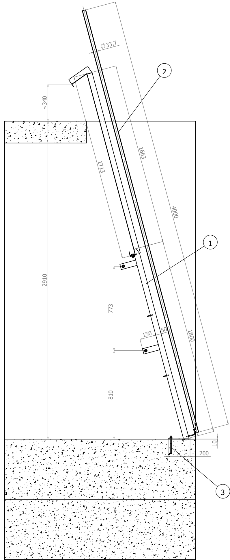
SECTION A-A
